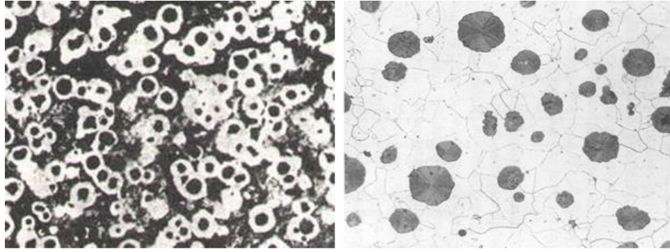
Şekil 2. 'Düktül Dökme Demir'in mikro yapısı.
