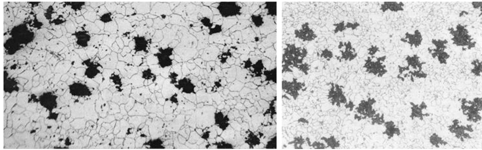
Şekil 3. 'Temper Dökme Demir ('malleable cast iron')'in mikro yapısı.
